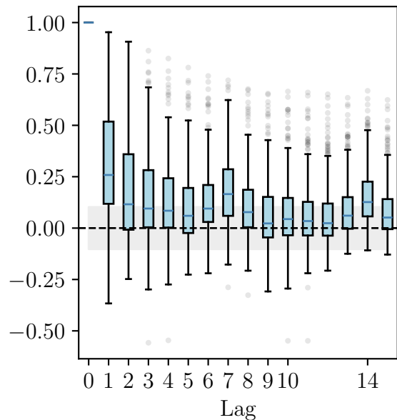
ACF
